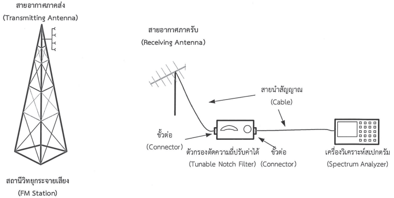
รูปที่ 2 ผังการต่อเครื่องมือสำหรับการทดสอบการแพร่แปลงปลอมผ่านสายอากาศ
