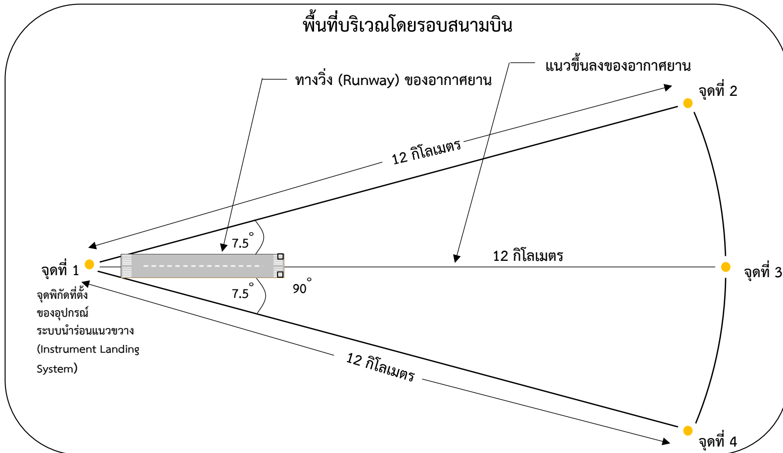
รูปที่ 1 พื้นที่ปลอดภัยรอบการใช้คลื่นความถี่สำหรับลดระดับเพดานบินและร่อนลงจอดของอากาศยาน หมายเหตุ อัตราส่วนของความยาวหรือมุมในรูปนี้ไม่ใช่มาตราส่วนย่อของขนาดจริง
